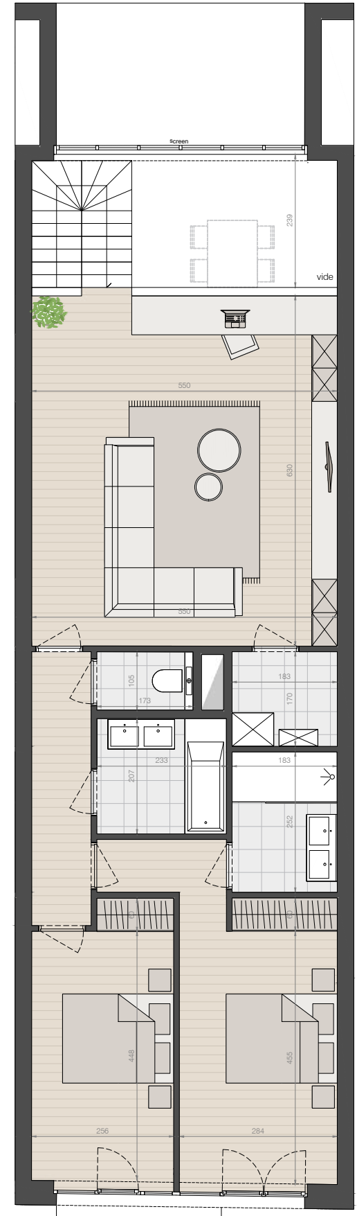
verdieping +2
